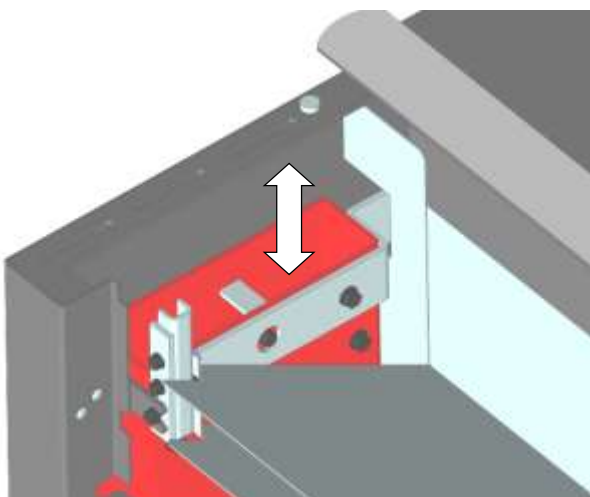
Abb. 58: Reinigung Heizgaszüge
