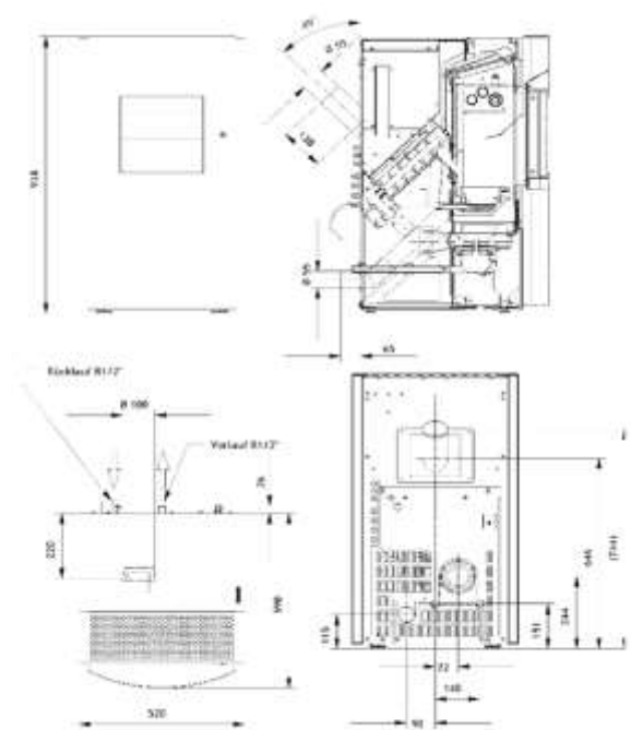
Abb. 98: Maßzeichnung "Frank" Waterplus
