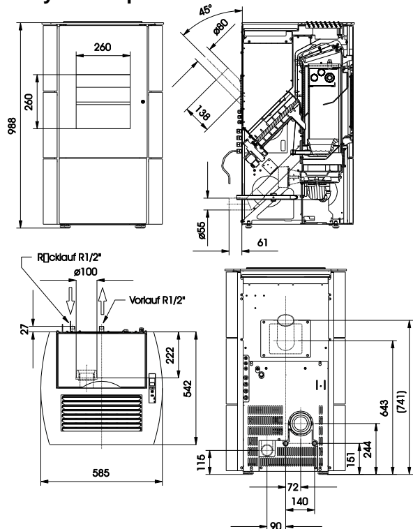
Abb. 104: Maßzeichnung "Ray" Waterplus
