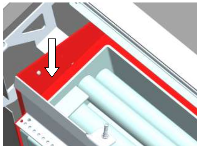
Abb. 72: Reinigung rechter Heizgaszug
