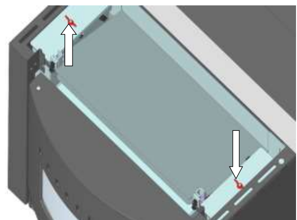
Abb. 56: Demontage Abdeckungen Heizgaszüge
