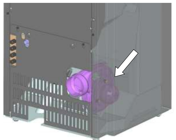
Abb. 67: Position Rauchgasgebläse
