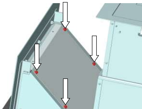
Abb. 40: Demontage Abdeckung PE
