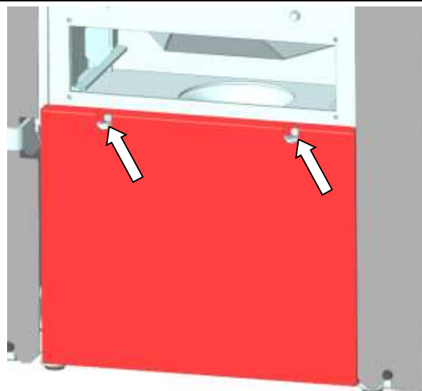
Abb. 80: Demontage Verkleidungsschürze
