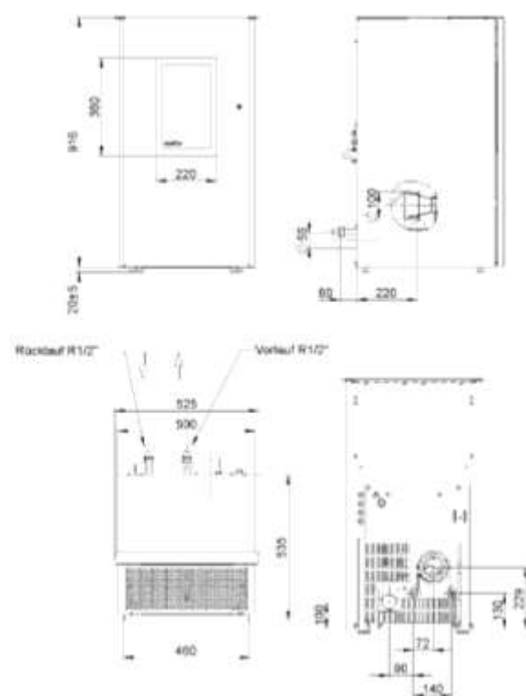
Abb. 100: Maßzeichnung "Pat" Waterplus
