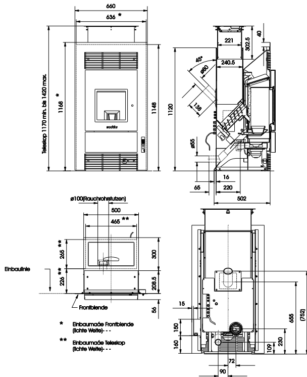
Abb. 101: Maßzeichnung "PE" SX
