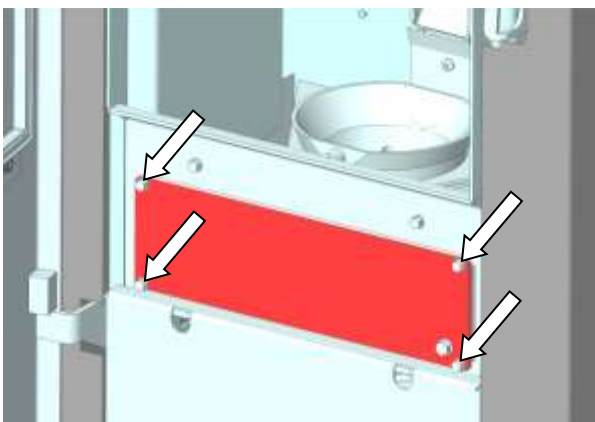
Abb. 74: Demontage Revisionsdeckel
