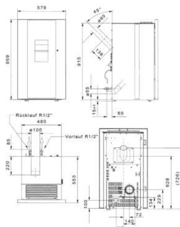
Abb. 94: Maßzeichnung "Dave" Waterplus
