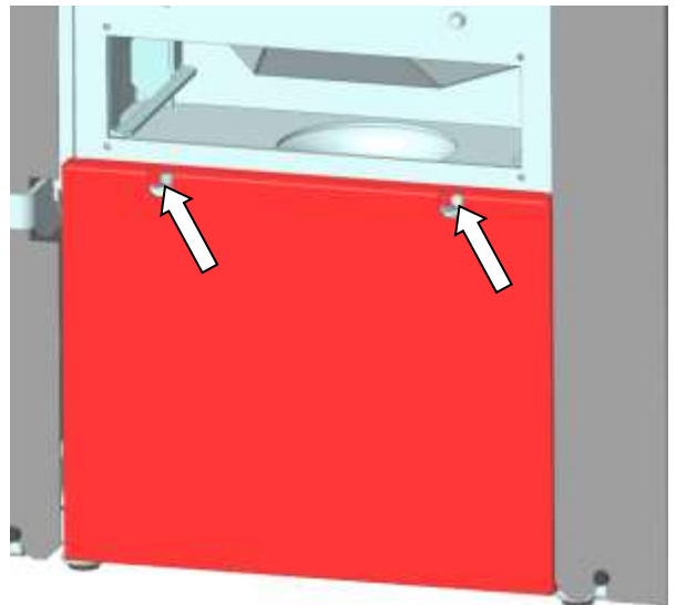
Abb. 51: Demontage Verkleidungsschürze
