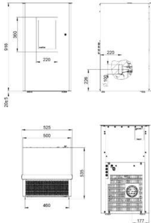
Abb. 99: Maßzeichnung "Pat" Airplus
