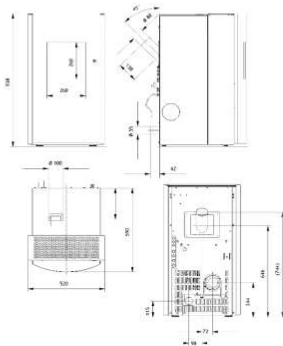
Abb. 97: Maßzeichnung "Frank" Airplus
