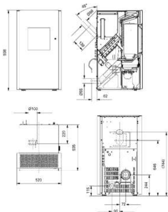
Abb. 95: Maßzeichnung "Frank" Airplus
