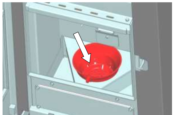
Abb. 46: Reinigung Brennertopf
