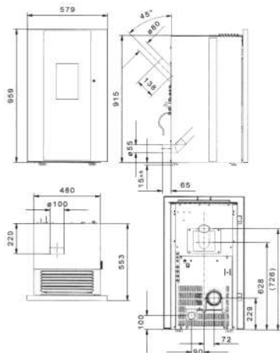
Abb. 93: Maßzeichnung "Dave" Airplus
