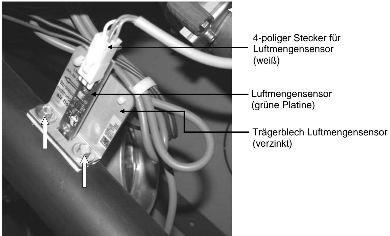
Abb. 89: Luftmengensensor
