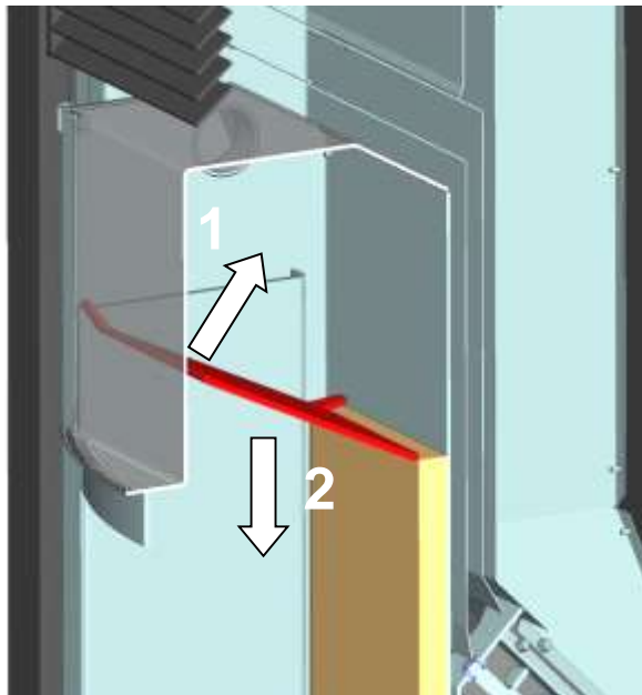
Abb. 52: Entnahme vordere Umlenkplatte
