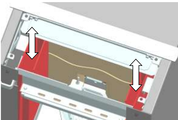
Abb. 44: Reinigung Heizgaszüge
