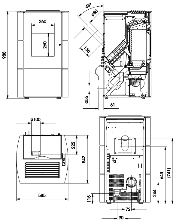
Abb. 103: Maßzeichnung "Ray" SX
