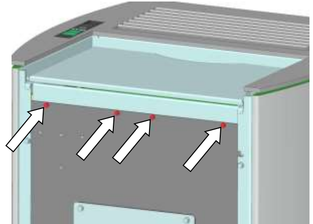
Abb. 38: Demontage Deckel
