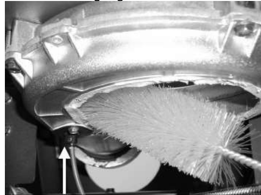
Abb. 83: Position Rauchgasfühler
