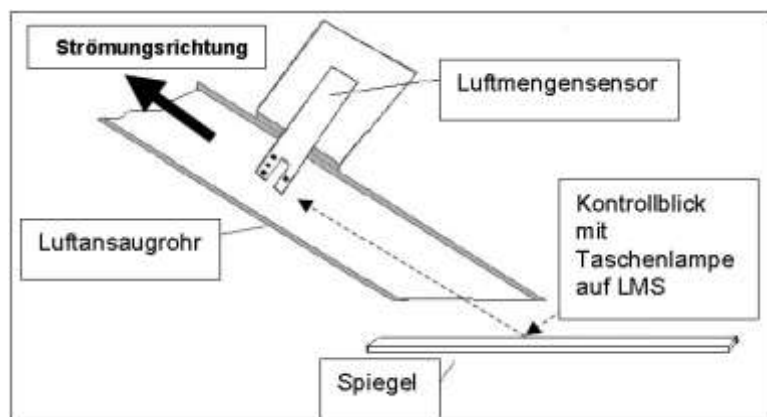
Abb. 85: Funktionsskizze Luftmengensensor
