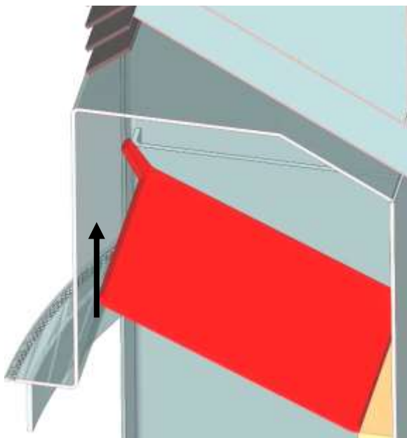
Abb. 53: Durchbrandschlitz Umlenkplatte
