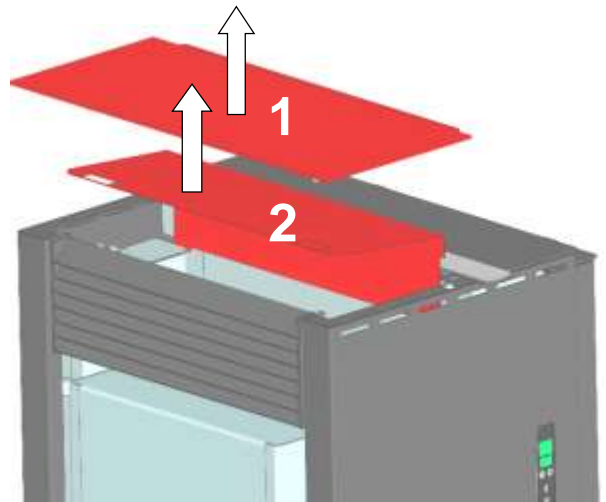
Abb. 54: Demontage Deckel und oberes Strahlungsschutzblech
