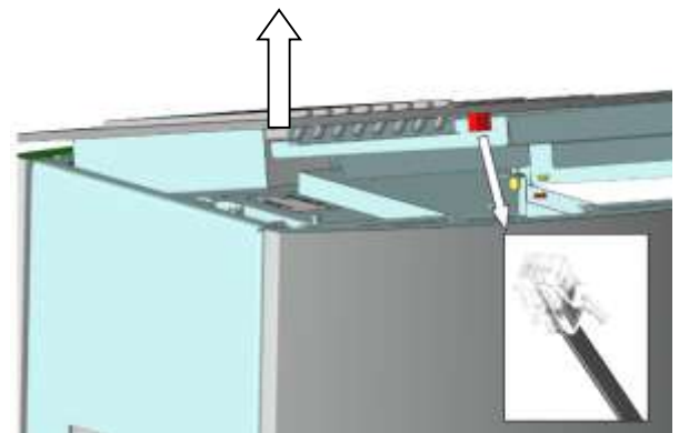
Abb. 39: Lösen Kabel Bedienboard
