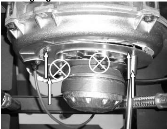
Abb. 81: Demontage Gebläsemotor
