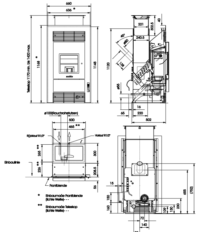
Abb. 102: Maßzeichnung "PE" Waterplus
