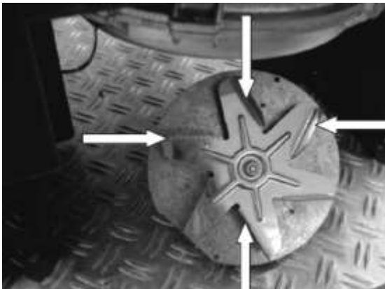
Abb. 82: Flügelrad Gebläse
