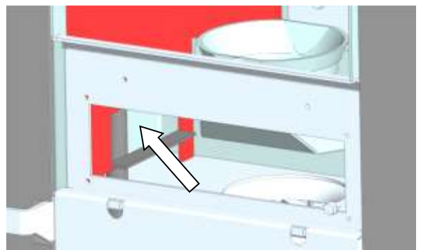
Abb. 78: Reinigung Heizgaszüge unten links
